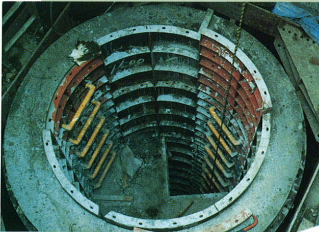
■二方向足掛同時打型枠
