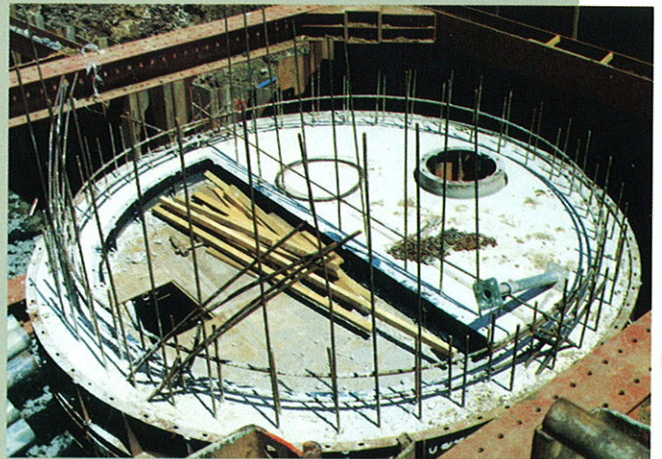
■スラブ開口部
