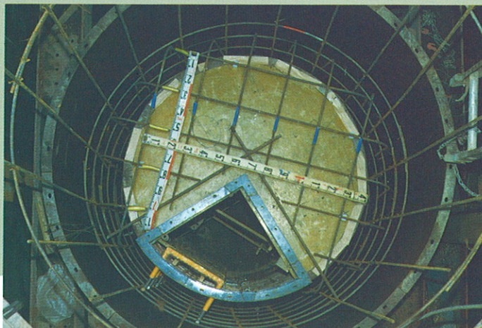
■2号人孔スラブ同時打型枠
