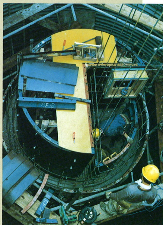
変則仕切壁型枠
