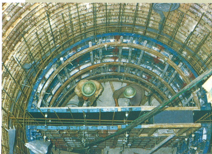
標準仕切壁
