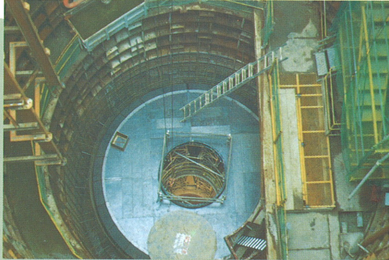
φ8,000 スラブハンチ型枠
