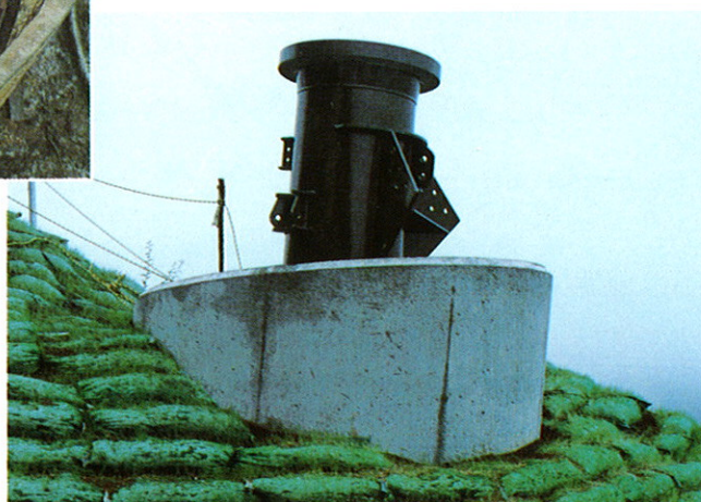
VI型基礎
